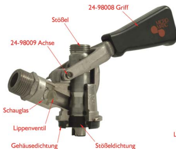
Kellerverbinder Typ A/M
