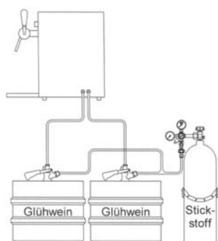
Heißgetränkzapfanlage OTHG 105
