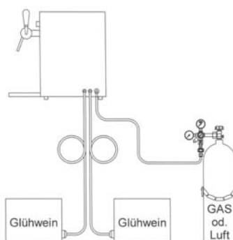
Heißgetränkzapfanlage OTHG 105-P mit integrierten Pumpen
